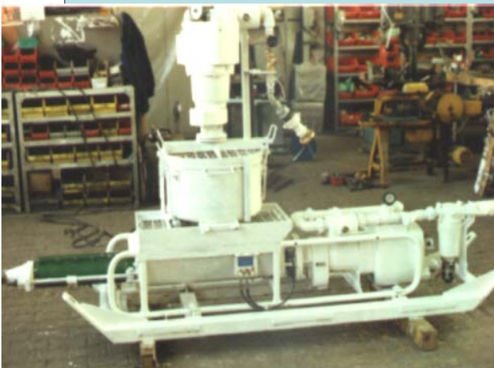
Mörtelpumpe und Tellermischer für Spezialmörtel zum Verankern, Injizieren und Hinterfüllen
